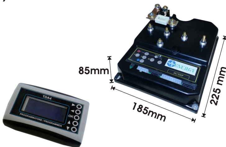
Calibratore TDA4 TDA4 Calibrator
